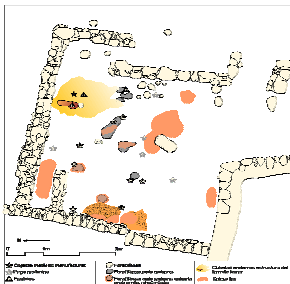
Estructures i distribució dels materials arqueològics del taller metal·lúrgic, s. I aC. Àmbit II, zona 1, Serrat dels Tres Hereus.
