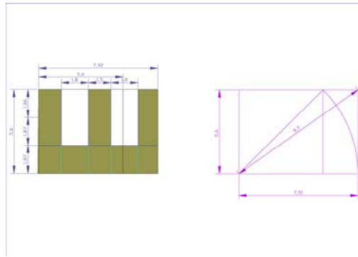
Torre YZ del poblat ibèric d'Alorda Park (Calafell, Baix Penedès) amb la proposada restitució modular i geomètrica.
