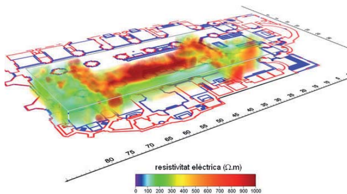
Mapa de resistivitat elèctrica obtingut de les prospeccions geofísiques dutes a terme a la Catedral de Tarragona.
