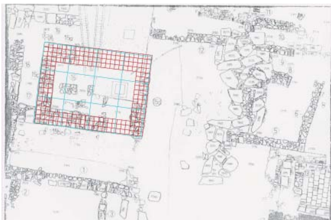
Torrassa del Grau Vell de Sagunt del segle II aC, amb superposició d'una graella basada en un pes oscus de 0,275 metres, a partir d'un rectangle de proporcions 3-4-5.
