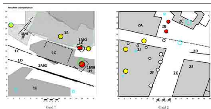
Esquema interpretatiu Grid 1 y 2. Geofísica CCS
